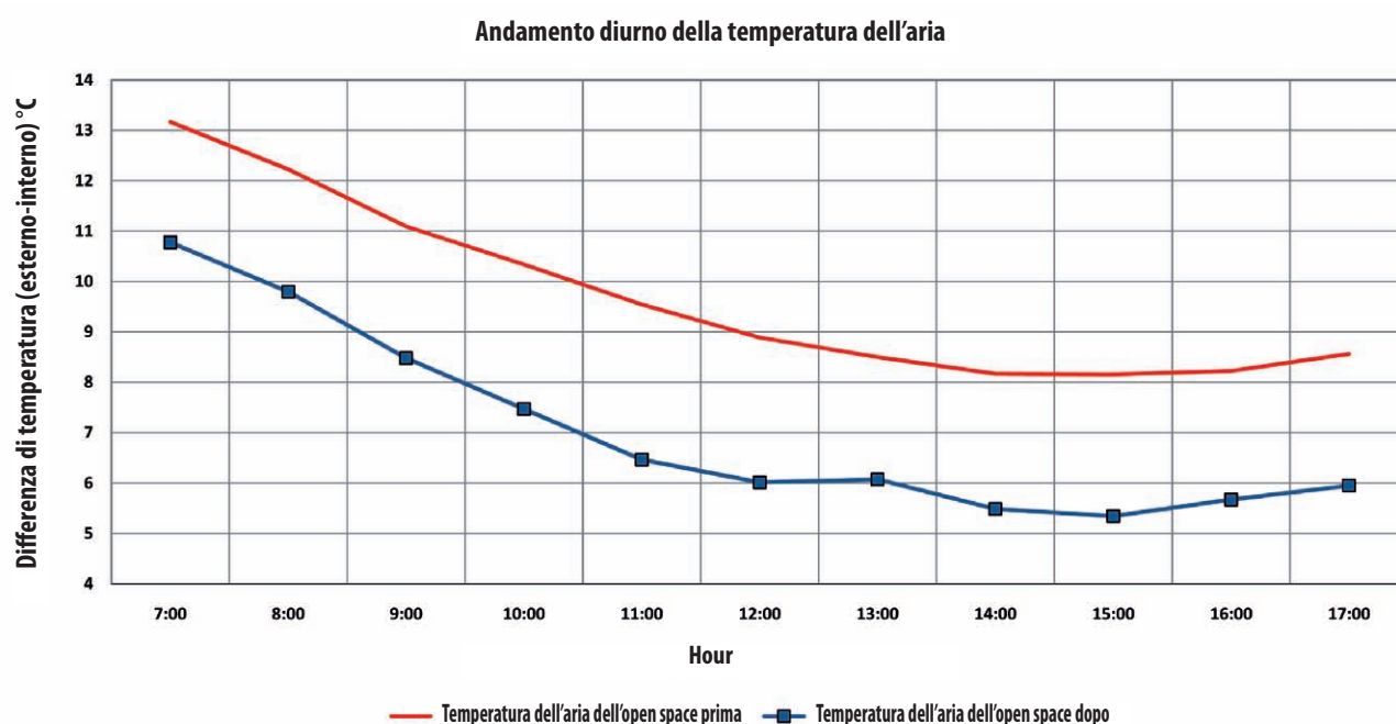
Figura 19. Andamento giornaliero della temperatura dell'aria misurata (differenze esterno-interno), prima e dopo l'applicazione dei materiali Cool Roofs
