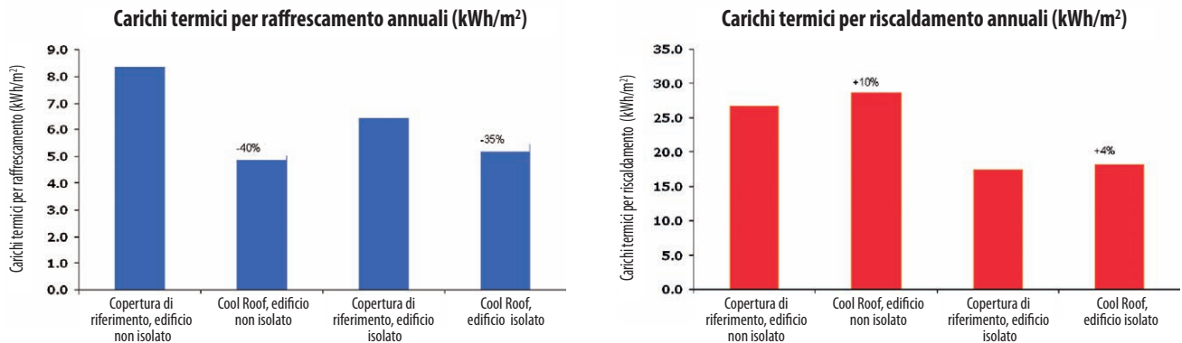
Figura 7. Carichi annuali di riscaldamento e raffreddamento (per l'edificio attuale non isolato e per lo stesso nell'ipotesi di un maggior isolamento)
