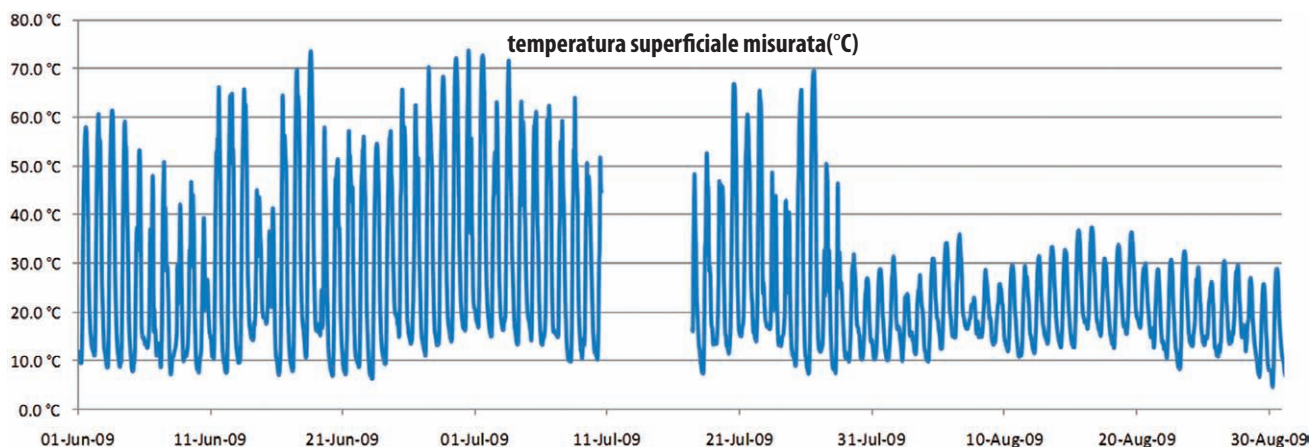
Figura 3. Temperatura superficiale prima e dopo l'applicazione del Cool Roof
