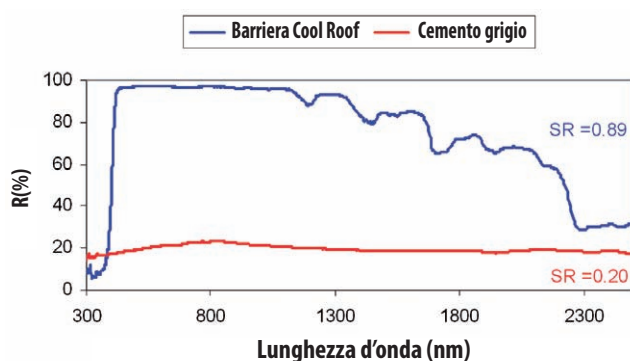
Figura 6. Riflettanza spettrale della superficie della copertura prima (cemento grigio, SR=0.2) e dopo l'applicazione del Cool Roof (ABOLIN Cool Roof barrier, SR=0.89)
