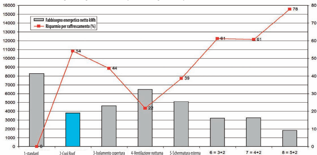
Fabbisogno energetico [kWh] e risparmio energetico [%] per l'edificio standard e le sue varianti
