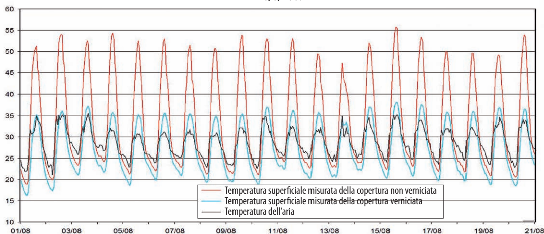
Figura 15. Confronto tra le temperature superficiali del Cool roof e della copertura originale riferite ad Agosto 2009
