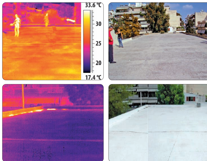
Figura 8. Immagini nel visibile e nell'infrarosso della superficie della copertura, mostrano le differenze di temperatura superficiali prima e dopo l'applicazione del Cool Roof
