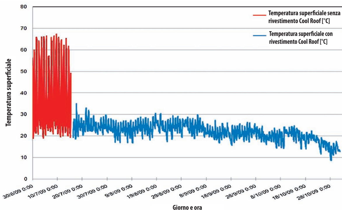
Figura 11. La temperatura superficiale della copertura prima e dopo l'applicazione del rivestimento Cool Roof
