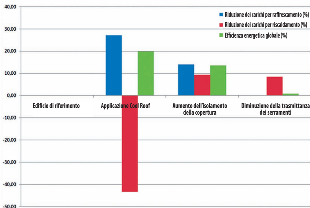
Figura 12. Confronto di diversi scenari di efficienza energetica
