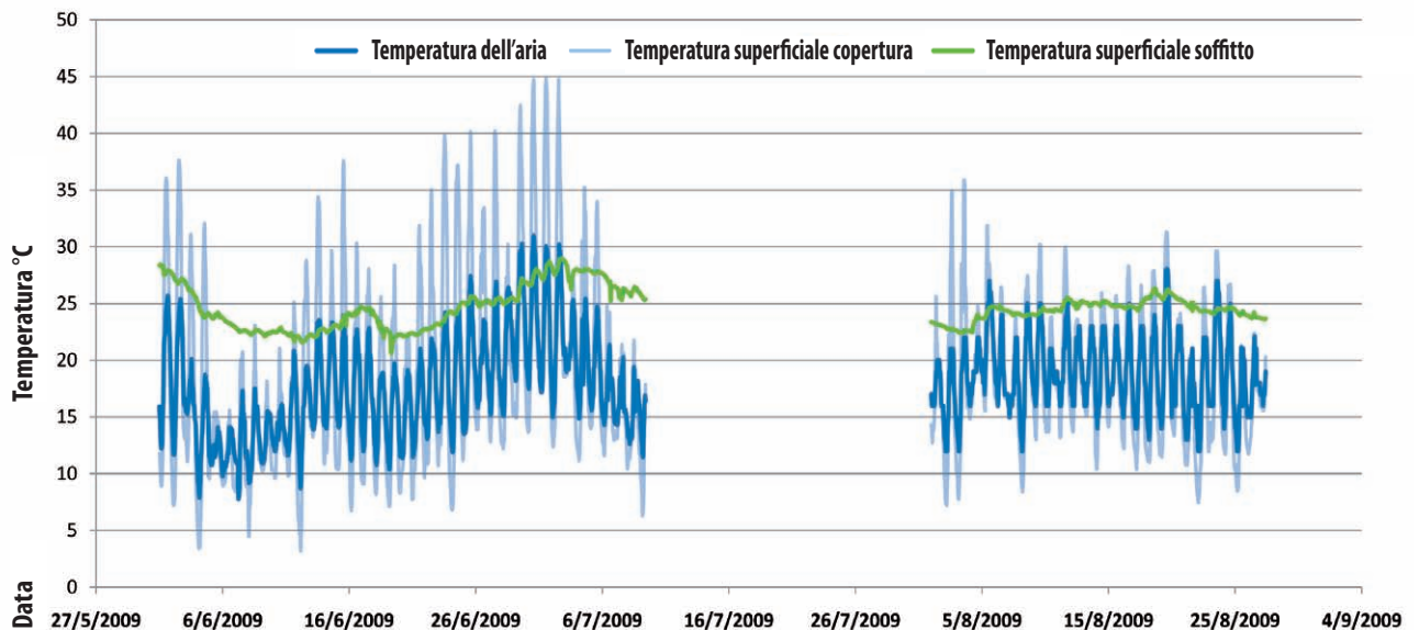
Figura 18. Temperature superficiali e dell'aria misurate prima e dopo l'applicazione del Cool Roof
