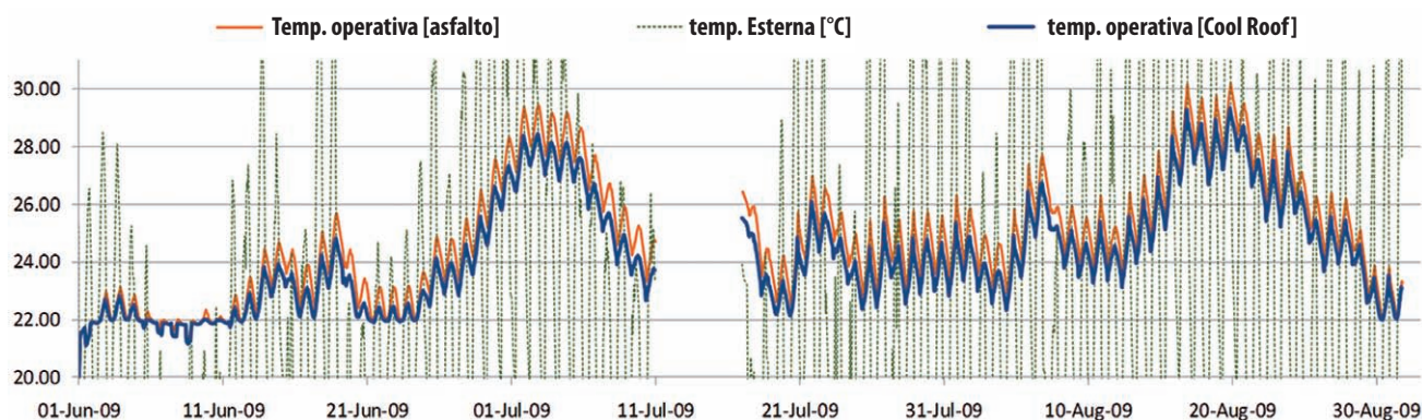
Figura 4. Andamento della Temperatura operativa prima e dopo l'applicazione del Cool Roof
